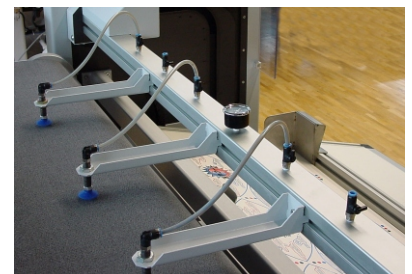
Individuell gesteuerte Saugteller sorgen für zuverlässigen Transport
